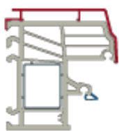
Standardblendrahmen für jeglichen Bauanschluss geeignet
