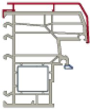
Standardblendrahmen für jeglichen Bauanschluss geeignet
